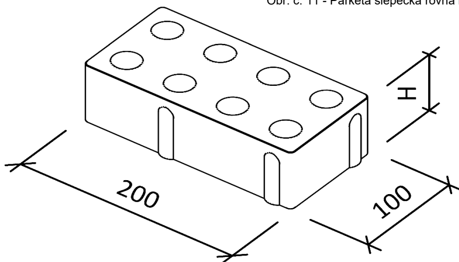
Obr. č. 11 - Parketa slepecká rovná hrana rozměry
