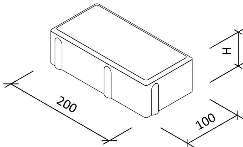
Obr. č. 10 - Parketa rovná hrana rozměry
