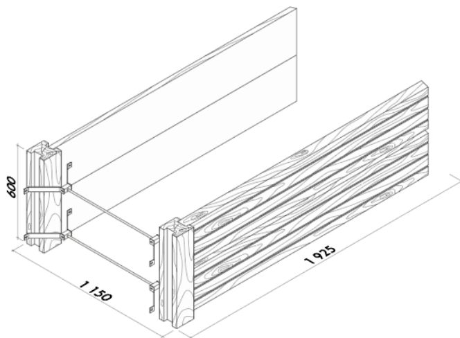
Obr. č. 15 – Prodlužovací set 60 rozměry
