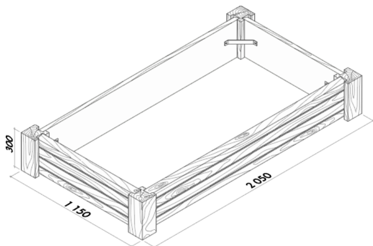
Obr. č. 12 – Zvýšený záhon 30 rozměry
