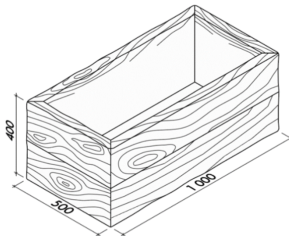
Obr. č. 10 – Květináč Elf rozměry
