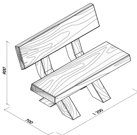
Obr. č. 16 – Lavice typ fošna s opěradlem 120
