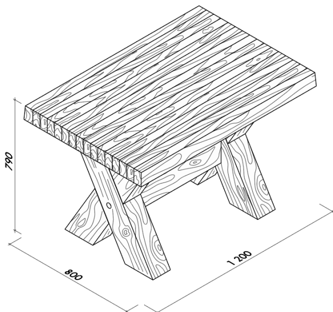
Obr. č. 18 – Stůl typ fošna 120
