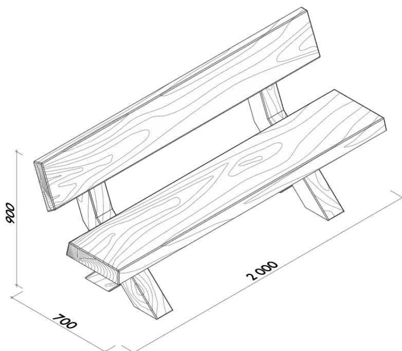
Obr. č. 13 – Lavice typ fošna 80 rozměry
