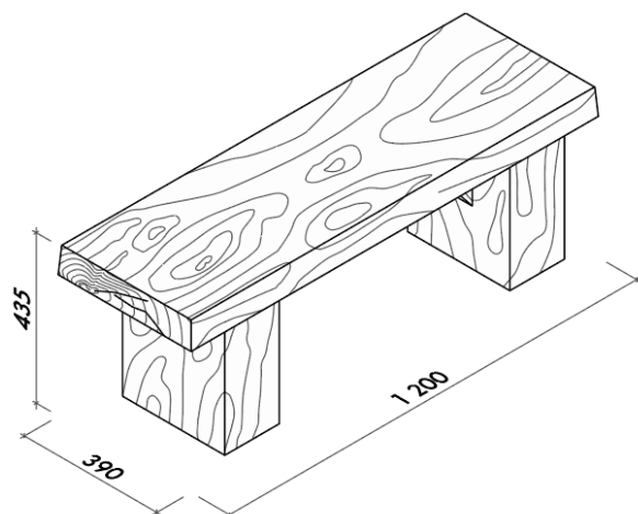
Obr. č. 15 – Lavice typ fošna 120 rozměry
