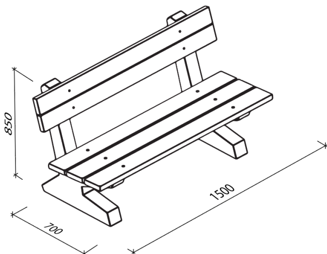
Obr. č. 3 Zahradní lavička s opěradlem - sedák dřevo
