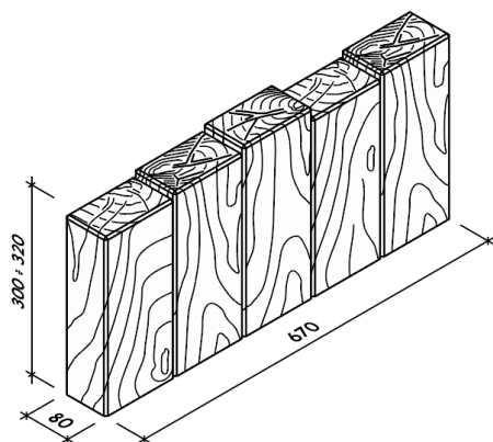
Obr. č. 7 – Palisádový obrubník – hranol rozměry
