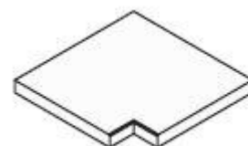
Obr. č. 2 - BAZÉNOVÝ LEM FANTASY – DESKOVÝ ostrý vnitřní roh 500 / 500 / 45
