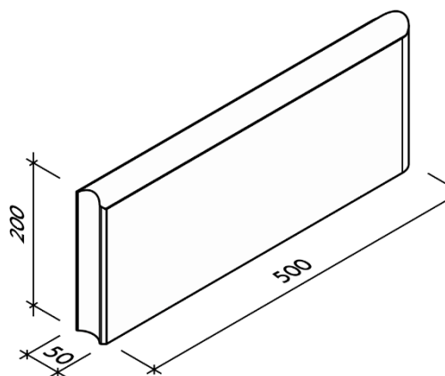
Obr. č. 15 Obrubník záhonový s kulatým zámkem 50 / 5 / 20 půlka
