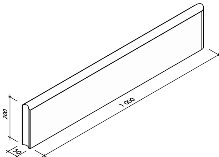
Obr. č. 16 Obrubník záhonový s kulatým zámkem 100 / 5 / 20
