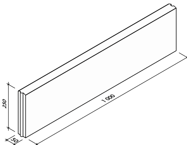
Obr. č. 14 Obrubník záhonový 100 / 5 / 25
