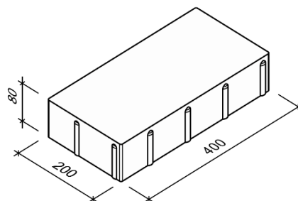
Obr. č. 5 – MILÁNO II. rozměry
