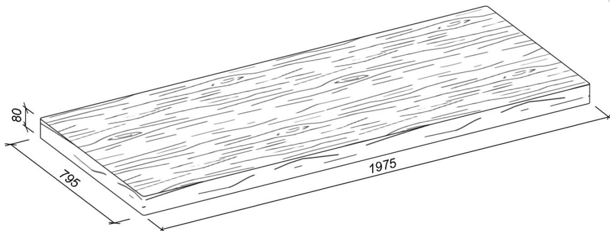
Obr. č. 15 – Podesta, šlapákové plato 200 / 80
