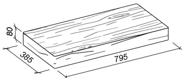
Obr. č. 10 – Schodišťová deska, šlapákové plato 80 / 40
