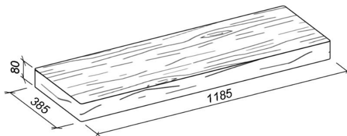
Obr. č. 11 – Schodišťová deska, šlapákové plato 120 / 40
