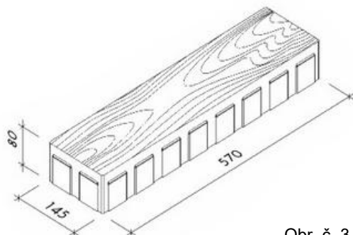
Obr. č. 3 – BOLZANO rozměry
