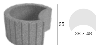
SVAHOVÁ TVÁRNICE DELTA VELKÁ Rozměry: 38 × 48 × 25 cm
