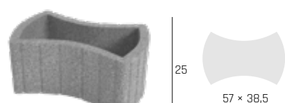
SVAHOVÁ TVÁRNICE OKTÁVA Rozměry: 57 × 38,5 × 25 cm
