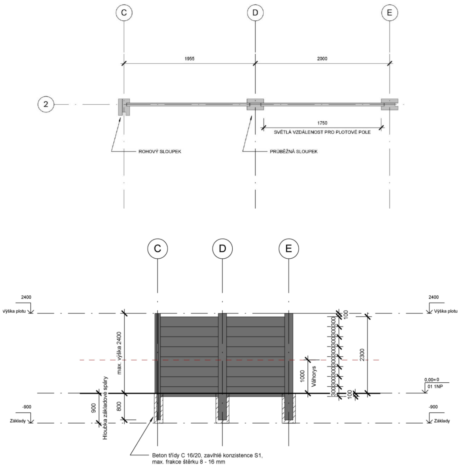
Obr. č. 7 – QUICK WALL WOOD – osová vzdálenost mezi jednotlivými sloupky
