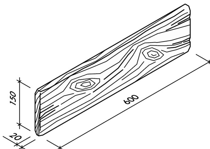
Obr. č. 4 – Obklad prkno rozměry
