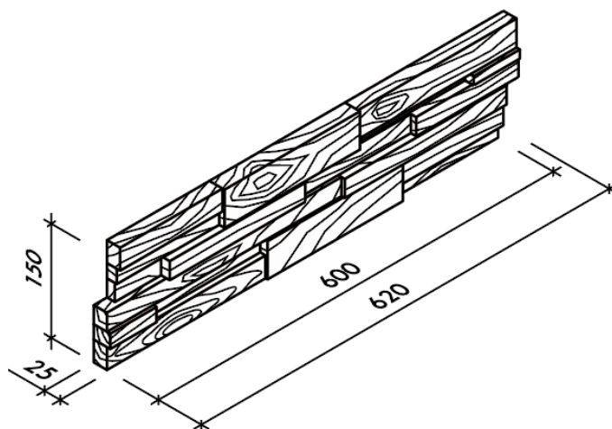
Obr. č. 5 – Obklad špalíky rozměry
