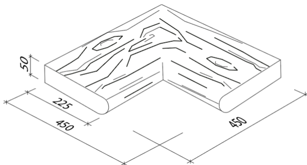
Obr. č. 5 – Bazénový lem vnitřní rohový – smrk
