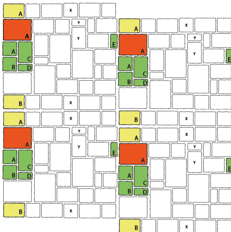
Obr. č. 2 – Rozložení kamenů ve čtyřech vrstvách na paletě
