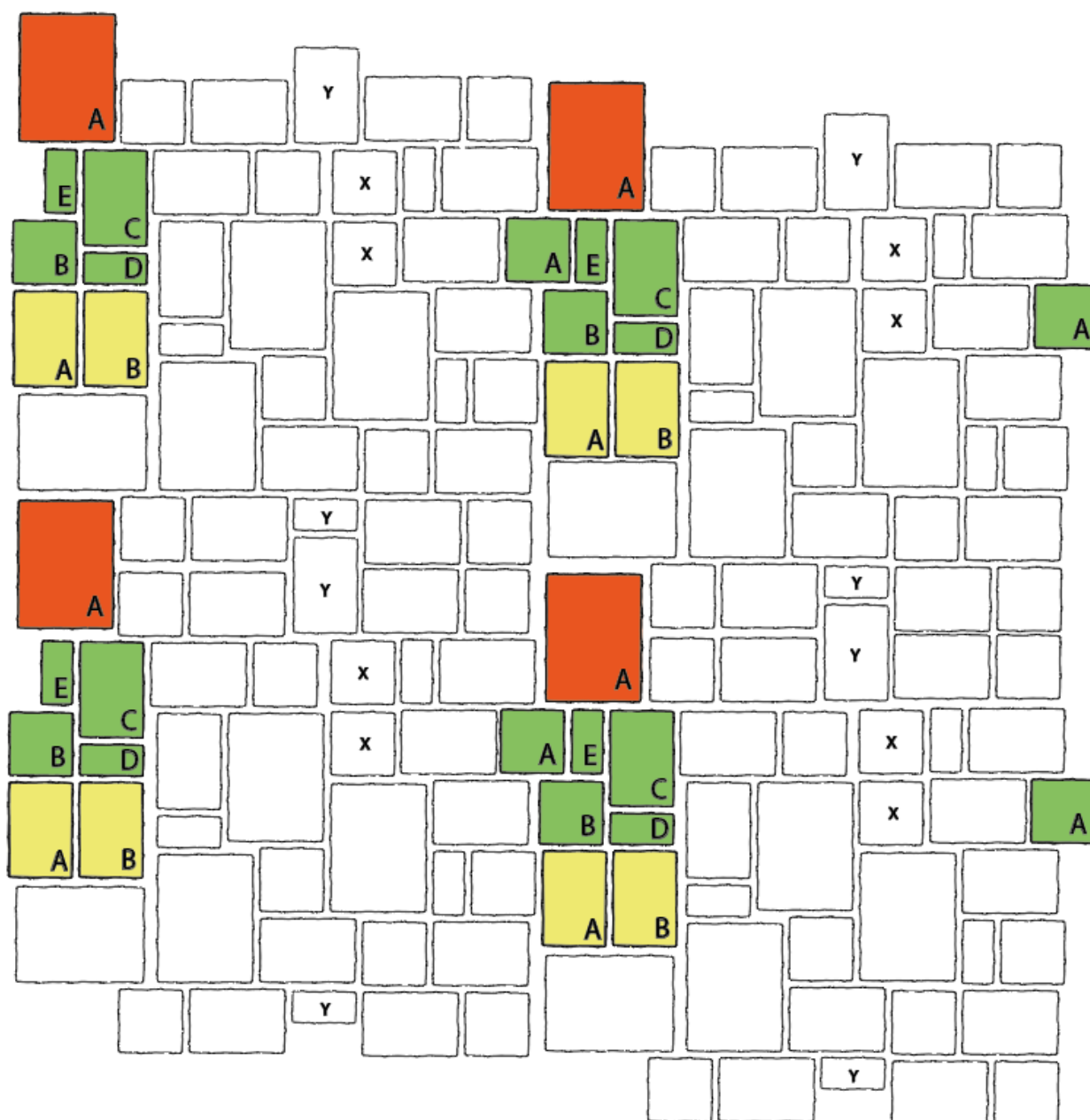
Obr. č. 3 – Rozložení čtyř vrstev s narušením krajních řad kamenů vrstvy
