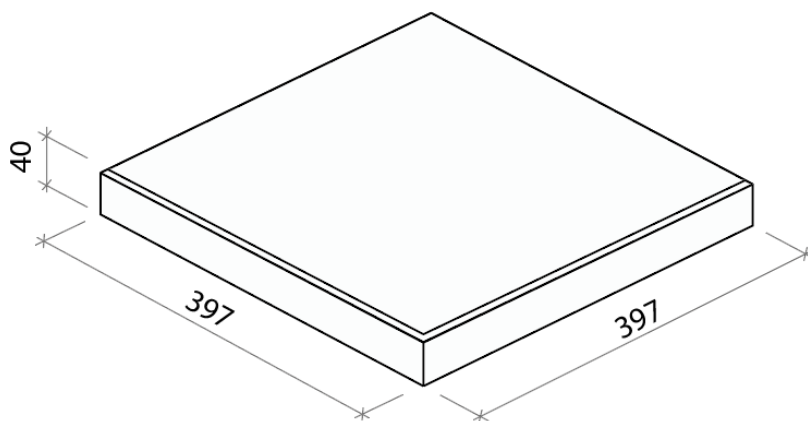
Obr. č. 2 – TYPICAL 40 / 40 / 4 rozměry
