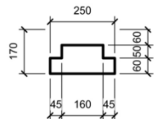
Obr. č.3 – QUICK WALL WOOD - sloupek dělený průběžný Dub výšky 210; 240; 270; 300; 320
