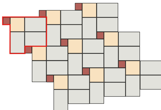
Skladba Plošná dlažba vymývaná 21
