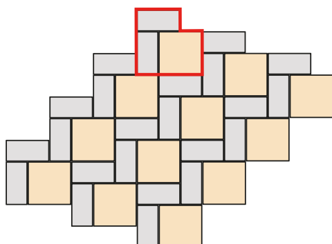
Skladba Plošná dlažba vymývaná 15
