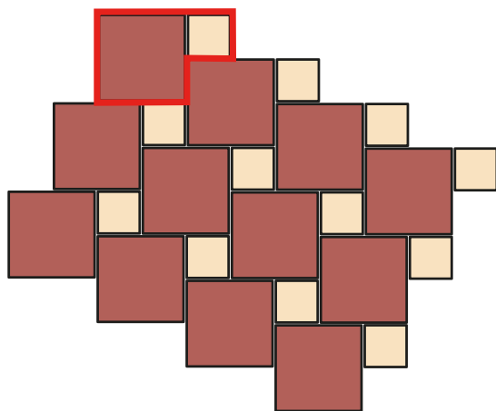
Skladba Plošná dlažba vymývaná 17
