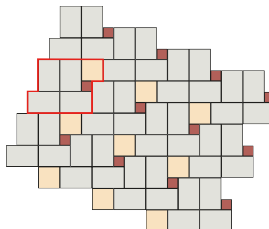
Skladba Plošná dlažba vymývaná 28
