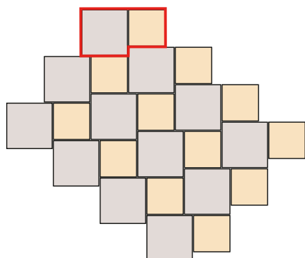
Skladba Plošná dlažba vymývaná 13
