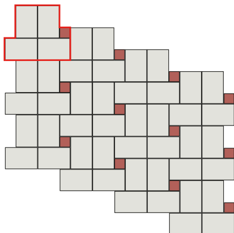
Skladba Plošná dlažba vymývaná 25
