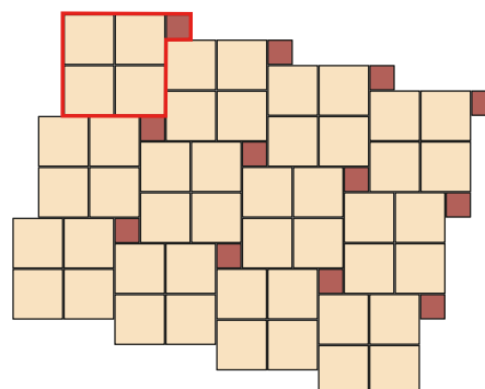
Skladba Plošná dlažba vymývaná 22
