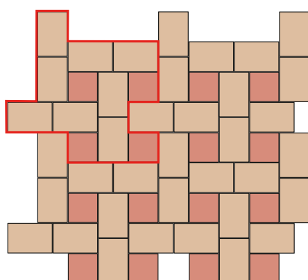
Skladba Plošná dlažba vymývaná 11
