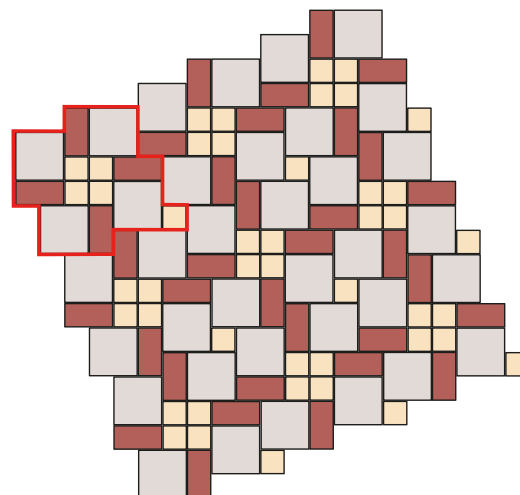
Skladba Plošná dlažba vymývaná 26
