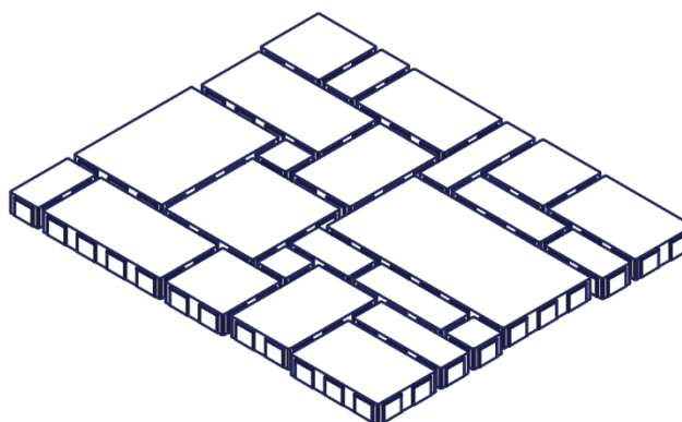
Obr. č.3 – Uložení prvků Kombi XL ve vrstvě na paletě varianta 1
