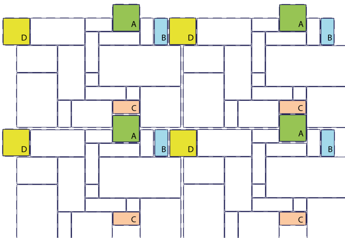
Obr. č.9 – Rozložení kamenů čtyř vrstev (po výměně kamenů)
