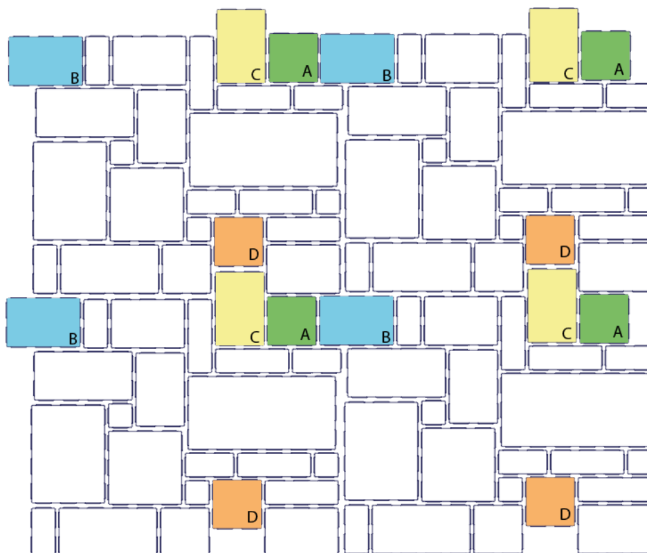
Obr. č.5 – Rozložení kamenů (po výměně kamenů) čtyř vrstev
