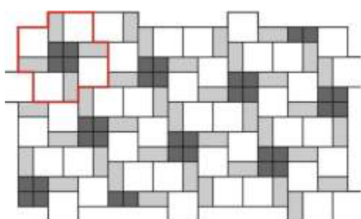
Obr. č.15 – Návrh pokládky z prvků Pl. Dlažba 40x40, Dek. pás 40x19,5 a Dekorační kostka 19,5x19,5
