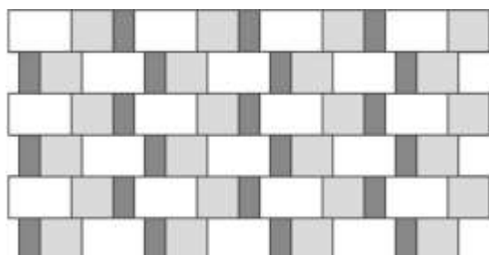
Obr. č.26 – Návrh pokládky z prvků Pl. Dlažba 60x40, Pl. Dlažba 40x40 a Dek. pás 40x19,5
