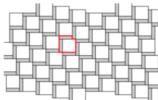
Obr. č.8 – Návrh pokládky z prvků Pl. Dlažba 40x40 a Dekorační pás 19,5x9,5
