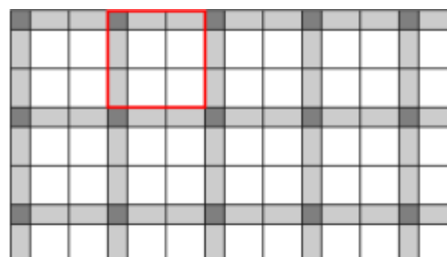
Obr. č.10 – Návrh pokládky z prvků Pl. Dlažba 40x40, Dekorační kostka 19,5x19,5 a Dekorační pás 40x19,5
