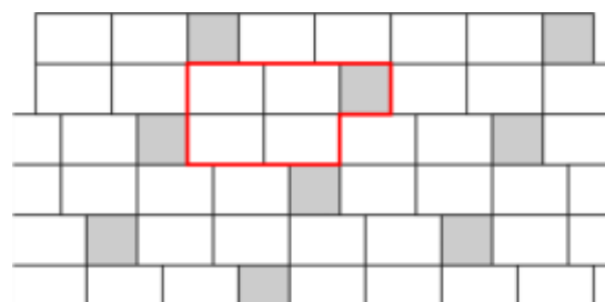
Obr. č.22 – Návrh pokládky z prvků Pl. Dlažba 60x40 a Pl. Dlažba 40x40
