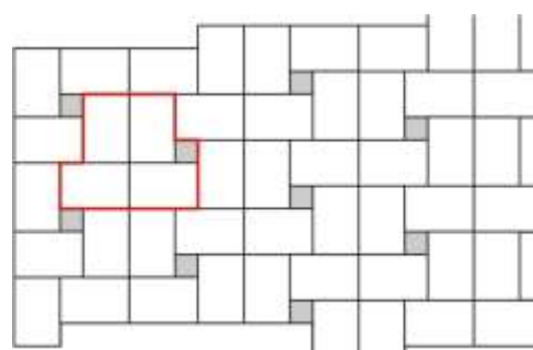
Obr. č.20 – Návrh pokládky z prvků Pl. Dlažba 60x40 a Dekorační kostka 19,5x19,5
