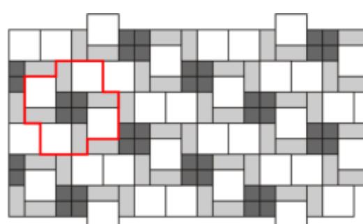
Obr. č.14 – Návrh pokládky z prvků Pl. Dlažba 40x40, Dekorační kostka 19,5x19,5 a Dekorační pás 40x19,5
