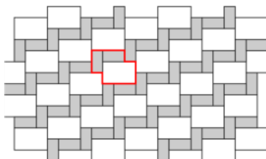
Obr. č.23 – Návrh pokládky z prvků Pl. Dlažba 60x40 a Dek. pás 40x19,5
