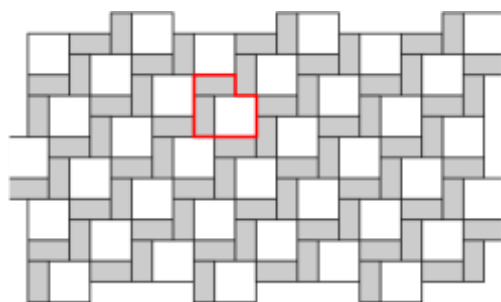
Obr. č.7 – Návrh pokládky z prvků Pl. Dlažba 40x40 a Dekorační pás 40x19,5
