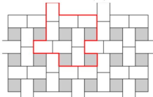
Obr. č.19 – Návrh pokládky z prvků Pl. Dlažba 60x40 a Pl. Dlažba 40x40
