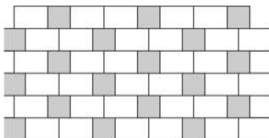
Obr. č.21 – Návrh pokládky z prvků Pl. Dlažba 60x40 a Pl. Dlažba 40x40
