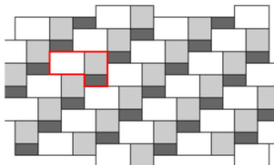
Obr. č.25 – Návrh pokládky z prvků Pl. Dlažba 60x40, Pl. Dlažba 40x40 a Dek. pás 40x19,5
