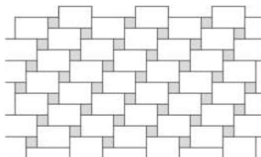
Obr. č.24 – Návrh pokládky z prvků Pl. Dlažba 60x40 a Dek. kostka 19,5x19,5
