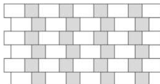
Obr. č.18 – Návrh pokládky z prvků Pl. Dlažba 60x40 a Pl. Dlažba 40x40
