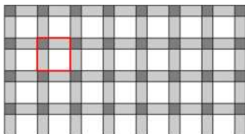
Obr. č.11 – Návrh pokládky z prvků Pl. Dlažba 40x40, Dekorační kostka 19,5x19,5 a Dekorační pás 40x19,5
