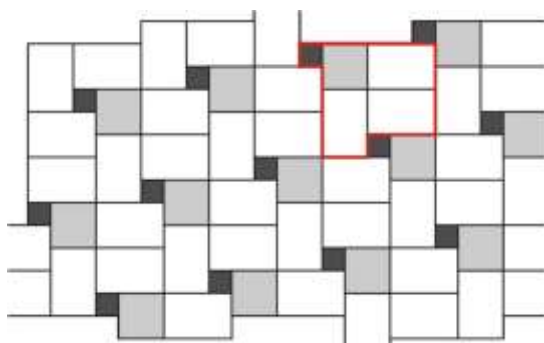
Obr. č.24 – Návrh pokládky z prvků Pl. Dlažba 60x40, Pl. Dlažba 40x40 a Dek. kostka 19,5x19,5
