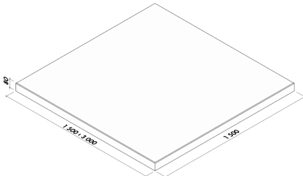
Obr. č.19 – Podestová deska Modern rozměry
