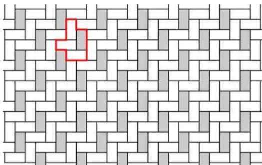
Obr. č.5 – Návrh pokládky z prvků Parketa
