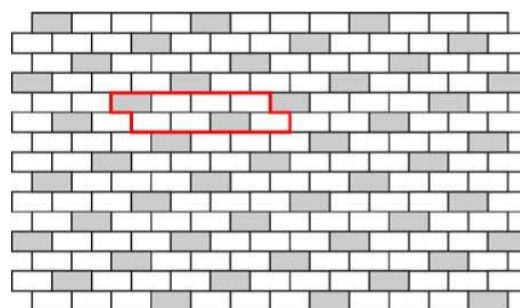
Obr. č.2 – Návrh pokládky z prvků Parketa
