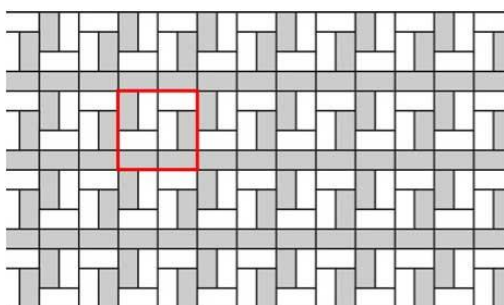
Obr. č.7 – Návrh pokládky z prvků Parketa
