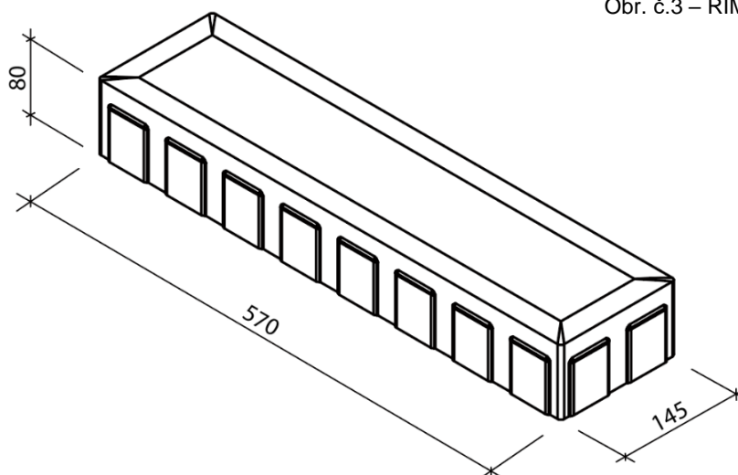
Obr. č.3 – RIMINI skladebné rozměry
