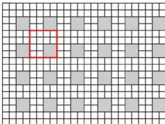
Obr. č.13 – Návrh pokládky z prvků Kostička 10x10 a Kostka 20x20
