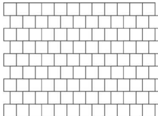
Obr. č.4 – Návrh pokládky z prvků Kostka 20x20
