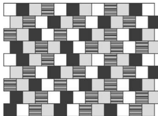
Obr. č.8 – Návrh pokládky z prvků Kostka 20x20
