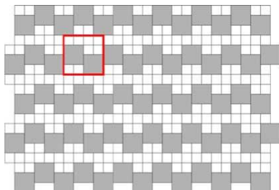
Obr. č.15 – Návrh pokládky z prvků Kostička 10x10 a Kostka 20x20
