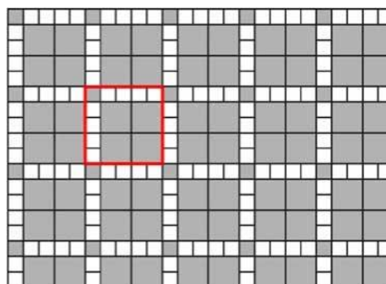
Obr. č.12 – Návrh pokládky z prvků Kostička 10x10 a Kostka 20x20
