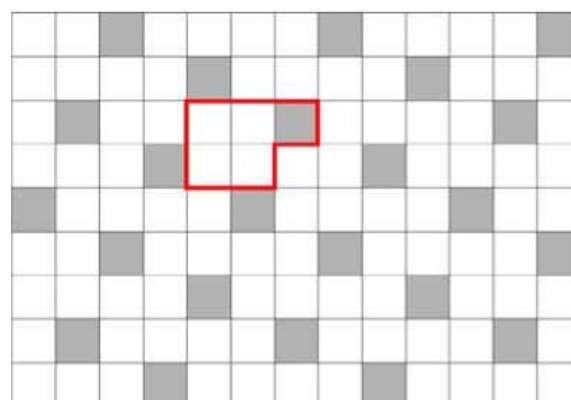
Obr. č.14 – Návrh pokládky z prvků Kostka 20x20
