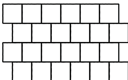
Obr. č.1 – Návrh pokládky z prvků Dlaždice Gabro 45 / 45
