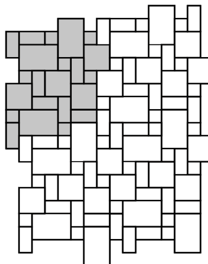
Obr. č.10 – Návrh pokládky z prvků Dlaždice Gabro 67,5 / 45, Dlaždice Gabro 45 / 45, Dlaždice Gabro 45 / 22,5 a Dlaždice Gabro 22,5 / 22,5
