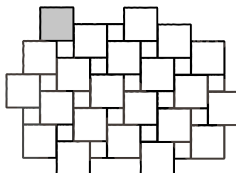
Obr. č.4 – Návrh pokládky z prvků Dlaždice Gabro 45 / 45 a Dlaždice Gabro 22,5 / 22,5
