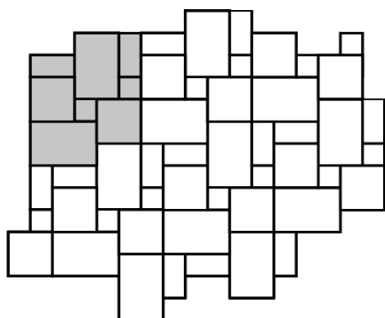
Obr. č.7 – Návrh pokládky z prvků Dlaždice Gabro 67,5 / 45, Dlaždice Gabro 45 / 45, Dlaždice Gabro 45 / 22,5 a Dlaždice Gabro 22,5 / 22,5
