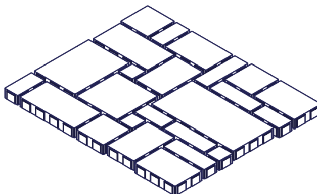
Obr. č.7 – Uložení prvků Kombi XL ve vrstvě na paletě varianta 2
