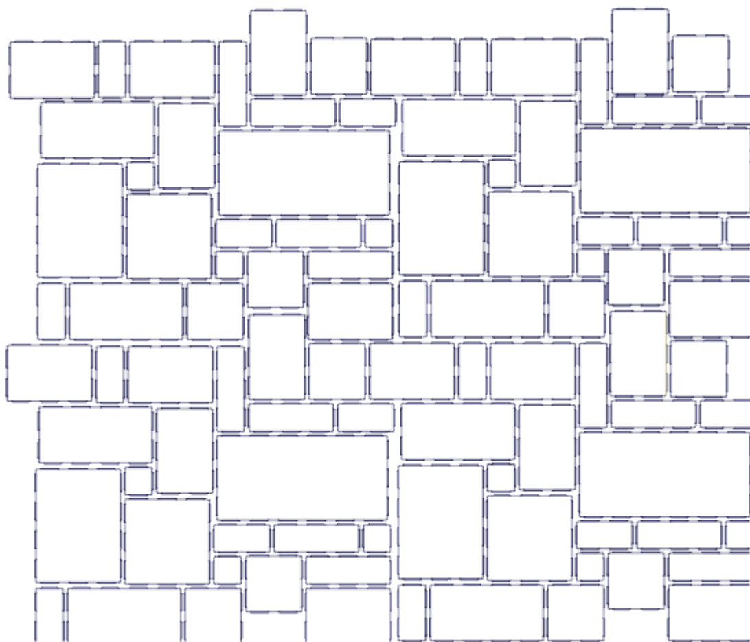
Obr. č.10 – Návrh pokládky varianta 2
