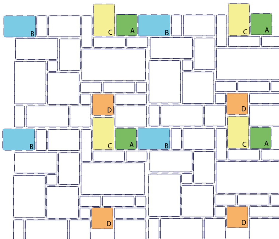
Obr. č.9 – Rozložení kamenů (po výměně kamenů) čtyř vrstev
