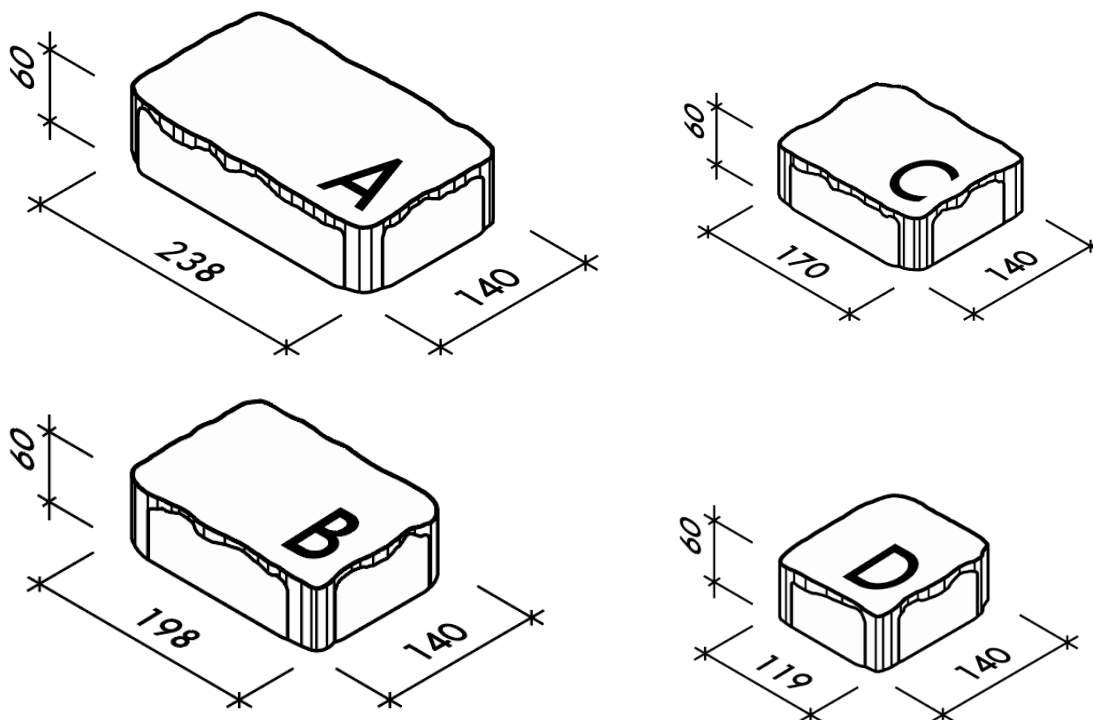
Obr. č.6 - RUSTIKO - rozměry
