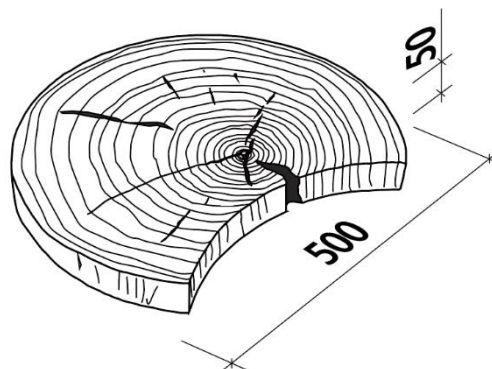
Obr. č.4 – VÝSEČ 50 rozměry
