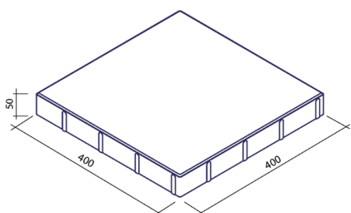
Obr. č.3 – DECENTO skladebné rozměry
