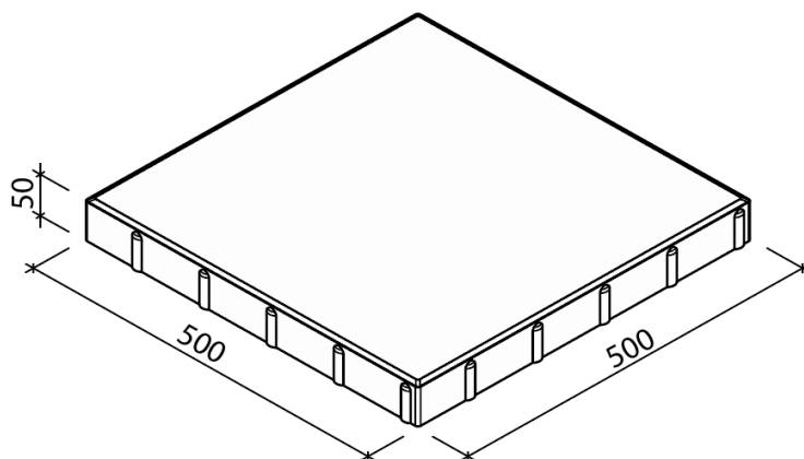
Obr. č.2 – GENEVA rozměry
