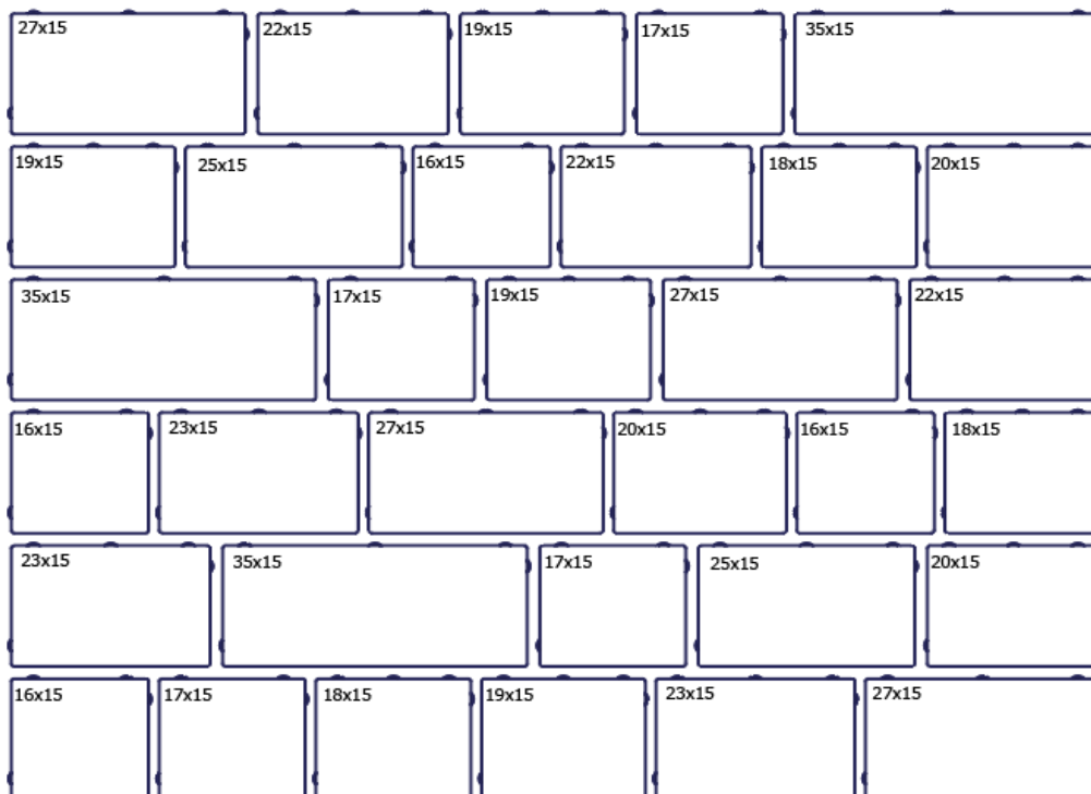
Obr. č.20 - PAVÉ II. - rozložení formátů na paletě (paletizace 2)
