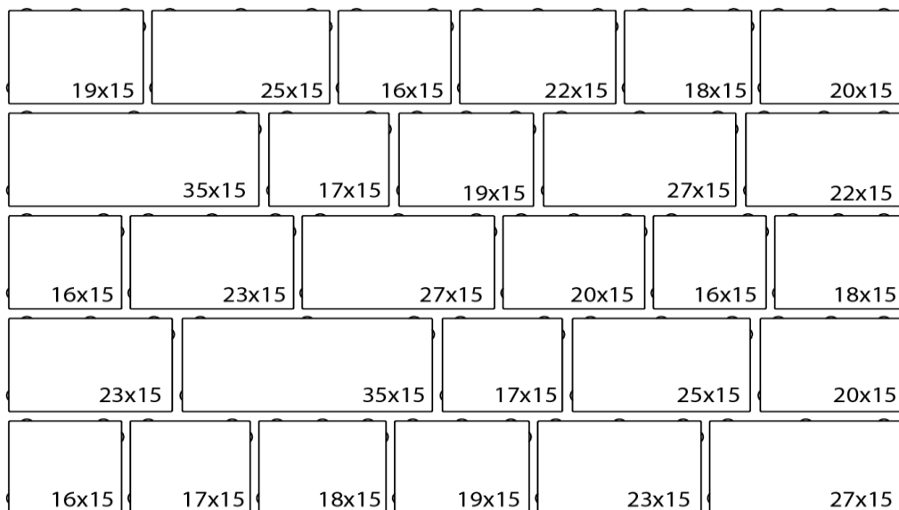
Obr. č.20 - PAVÉ II. - rozložení formátů na paletě (paletizace 2)
