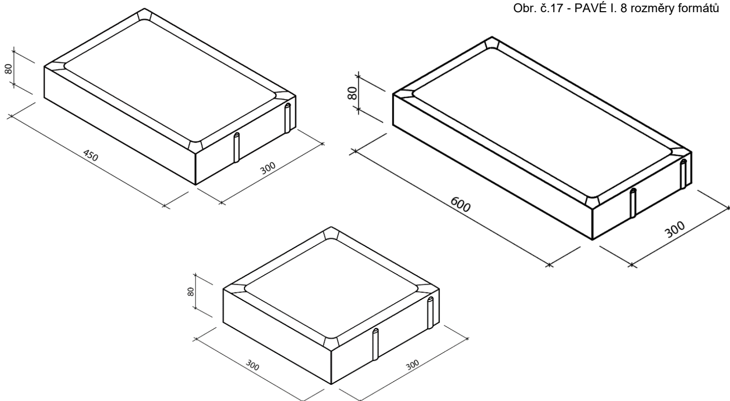
Obr. č.17 - PAVÉ I. 8 rozměry formátů
