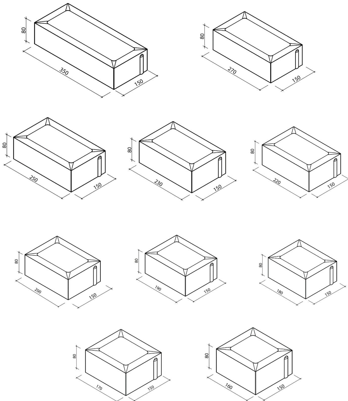
Obr. č.18 - PAVÉ II. 8 rozměry formátů
