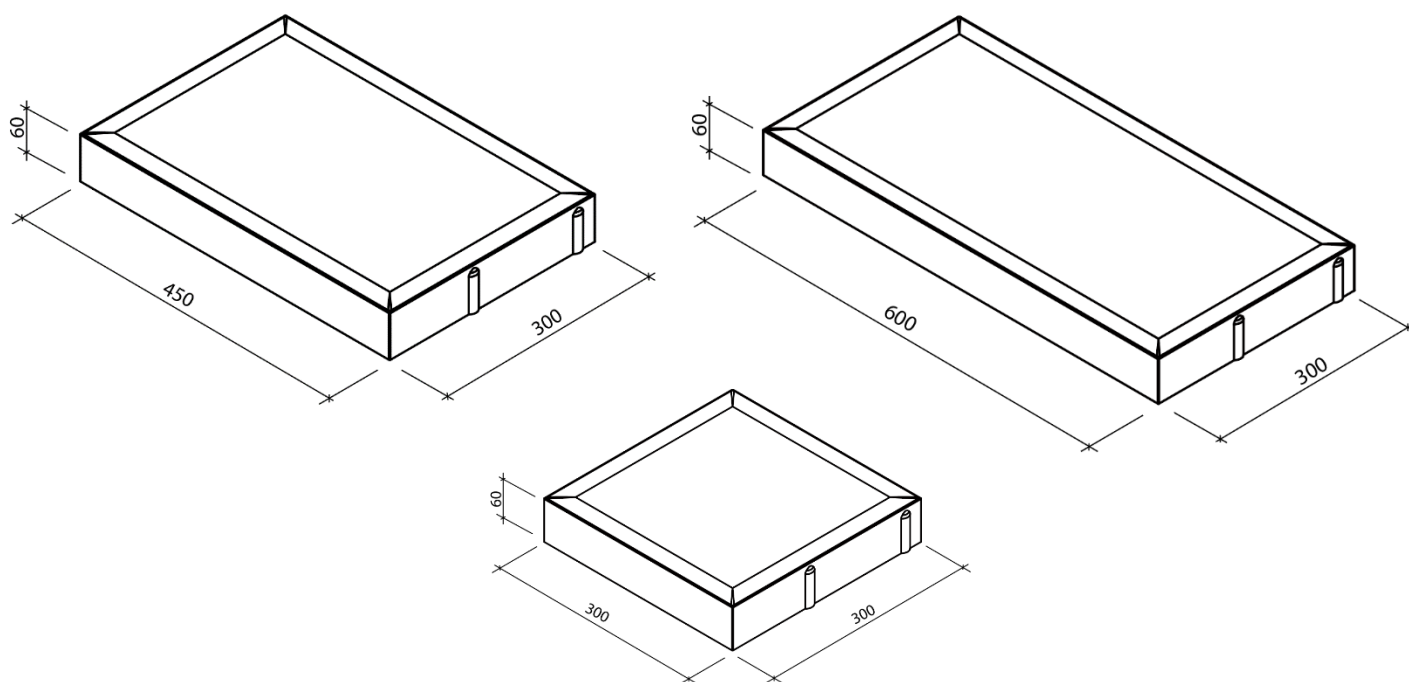
Obr. č.17 - PAVÉ I. 8 rozměry formátů
