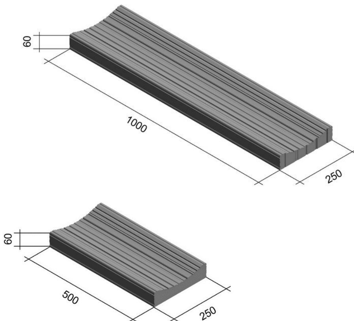
Obr. č.3 – ŽLAB MALÝ, ŽLAB VELKÝ rozměry
