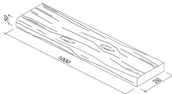
Obr. č.13 Bazénový lem přímý D1
