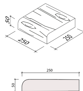
Obr. č.9 Bazénový lem přímý D4
