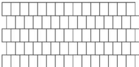
Obr. č.3 – Návrh pokládky z prvků Obdélník
