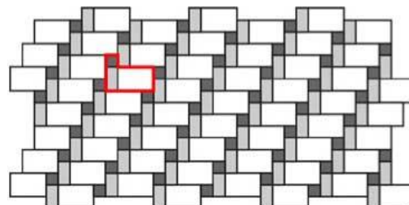
Obr. č.16 – Návrh pokládky z prvků Obdélník, Parketa a Kostička
