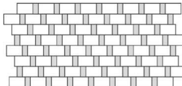
Obr. č.10 – Návrh pokládky z prvků Obdélník a Parketa
