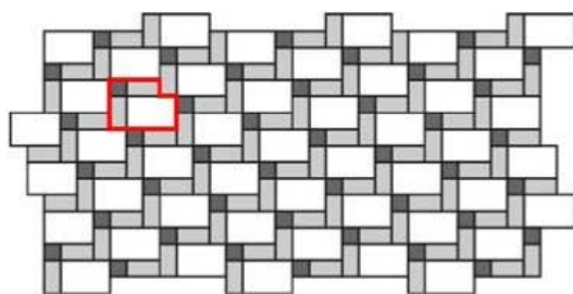
Obr. č.17 – Návrh pokládky z prvků Obdélník, Parketa a Kostička
