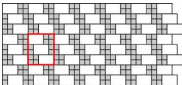
Obr. č.19 – Návrh pokládky z prvků Obdélník a Kostička
