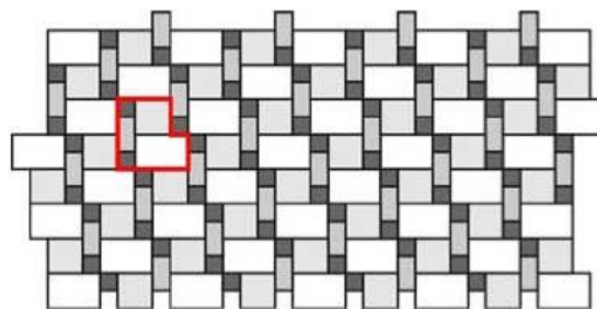
Obr. č.18 – Návrh pokládky z prvků Obdélník, Kostka, Parketa a Kostička
