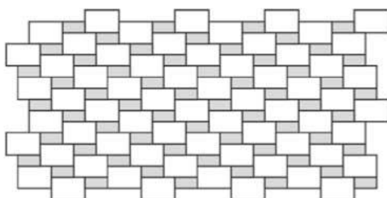
Obr. č.13 – Návrh pokládky z prvků Obdélník a Parketa
