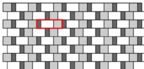
Obr. č.20 – Návrh pokládky z prvků Obdélník, Kostka a Parketa
