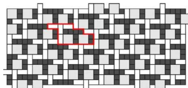
Obr. č.22 – Návrh pokládky z prvků Kostka 20x20, Kostička 10x10 a Parketa
