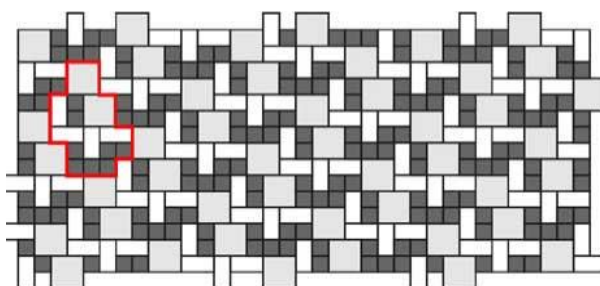
Obr. č.23 – Návrh pokládky z prvků Kostka 20x20, Kostička 10x10 a Parketa
