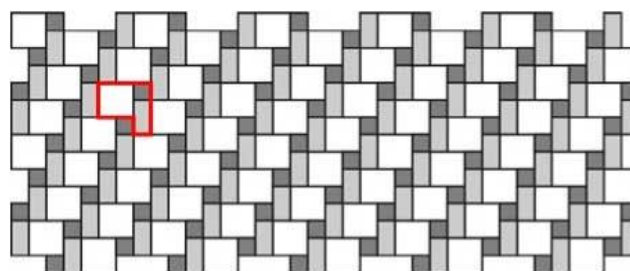
Obr. č.2 – Návrh pokládky z prvků Kostka 20x20, Kostička 10x10 a Parketa
