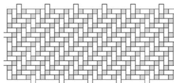
Obr. č.14 – Návrh pokládky z prvků Kostičkaka 10x10 a Parketa
