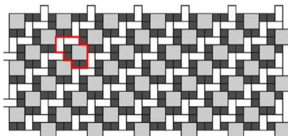
Obr. č.21 – Návrh pokládky z prvků Kostka 20x20, Kostička 10x10 a Parketa
