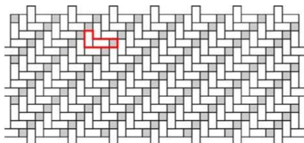
Obr. č.15 – Návrh pokládky z prvků Kostička 10x10 a Parketa
