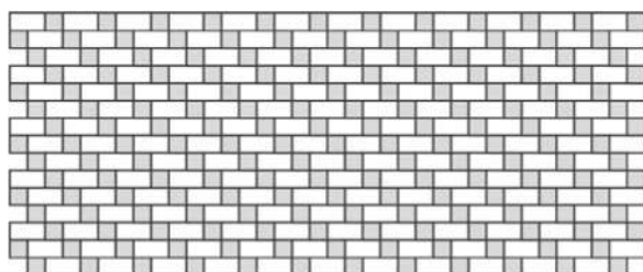
Obr. č.7 – Návrh pokládky z prvků Kostička 10x10 a Parketa
