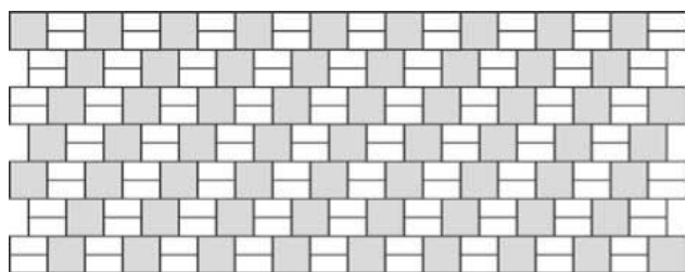
Obr. č.5 – Návrh pokládky z prvků Kostka 20x20 a Parketa
