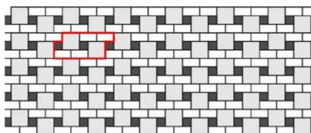
Obr. č.20 – Návrh pokládky z prvků Kostka 20x20, Kostička 10x10 a Parketa
