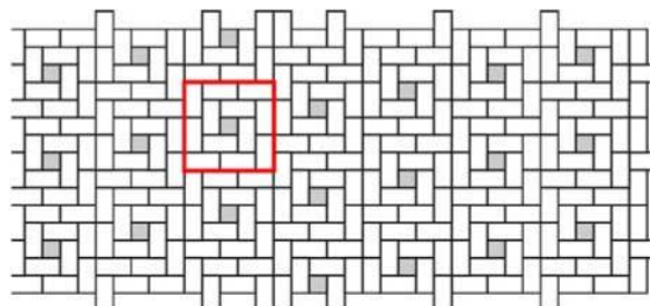
Obr. č.18 – Návrh pokládky z prvků Kostičkaka 10x10 a Parketa
