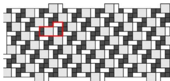
Obr. č.24 – Návrh pokládky z prvků Kostka 20x20, Kostička 10x10 a Parketa
