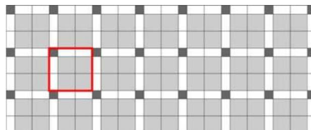
Obr. č.4 – Návrh pokládky z prvků Kostka 20x20, Kostička 10x10 a Parketa
