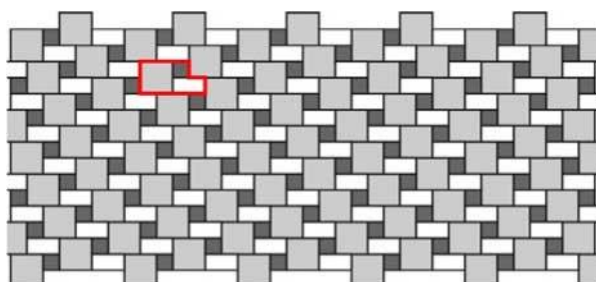
Obr. č.11 – Návrh pokládky z prvků Kostka 20x20, Kostička 10x10 a Parketa
