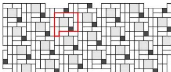
Obr. č.9 – Návrh pokládky z prvků Kostka 20x20, Kostička 10x10 a Parketa
