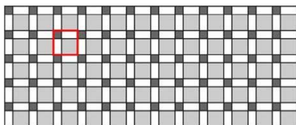
Obr. č.13 – Návrh pokládky z prvků Kostka 20x20, Kostička 10x10 a Parketa
