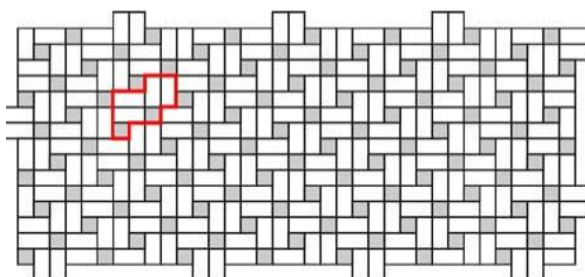
Obr. č.19 – Návrh pokládky z prvků Kostka 20x20 a Parketa
