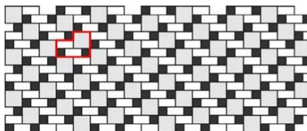
Obr. č.12 – Návrh pokládky z prvků Kostka 20x20, Kostička 10x10 a Parketa
