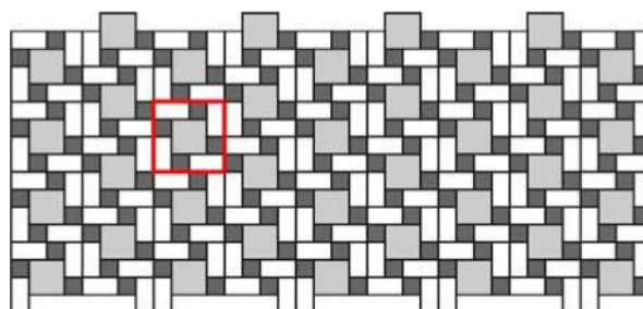
Obr. č.25 – Návrh pokládky z prvků Kostka 20x20, Kostička 10x10 a Parketa
