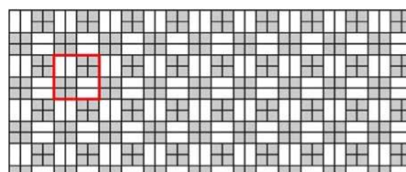
Obr. č.8 – Návrh pokládky z prvků Kostička 10x10 a Parketa
