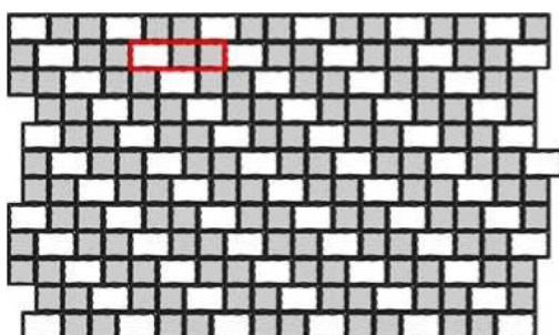
Obr. č.7 – Návrh pokládky z prvků Rocco II. a Rocco I.
