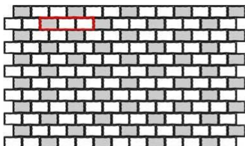
Obr. č.5 – Návrh pokládky z prvků Rocco II.
