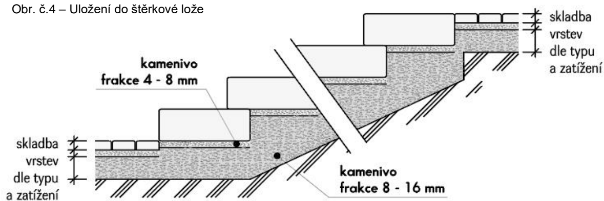
Obr. č.4 – Uložení do šterkové lože
