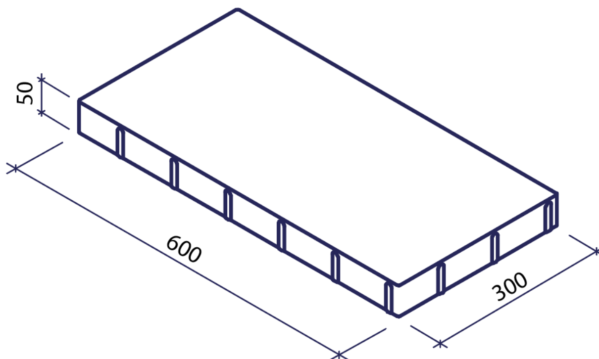
Obr. č.2 – STADIO rozměry
