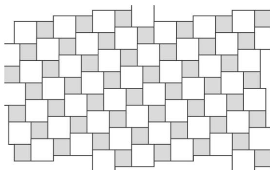
Obr. č.7 – Návrh pokládky z prvků Plošná dlažba 30x30 a 40x40
