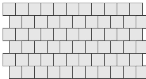
Obr. č.2 – Návrh pokládky z prvků Plošná dlažba 30x30
