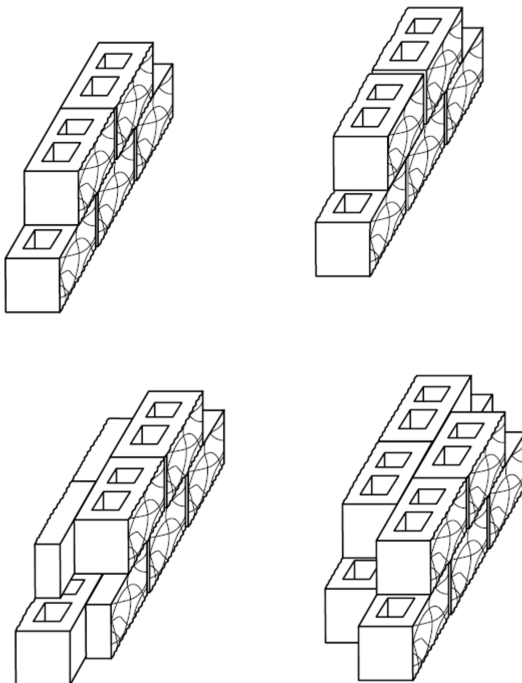
Obr. č.20 Vazba bloků ve zdivu
