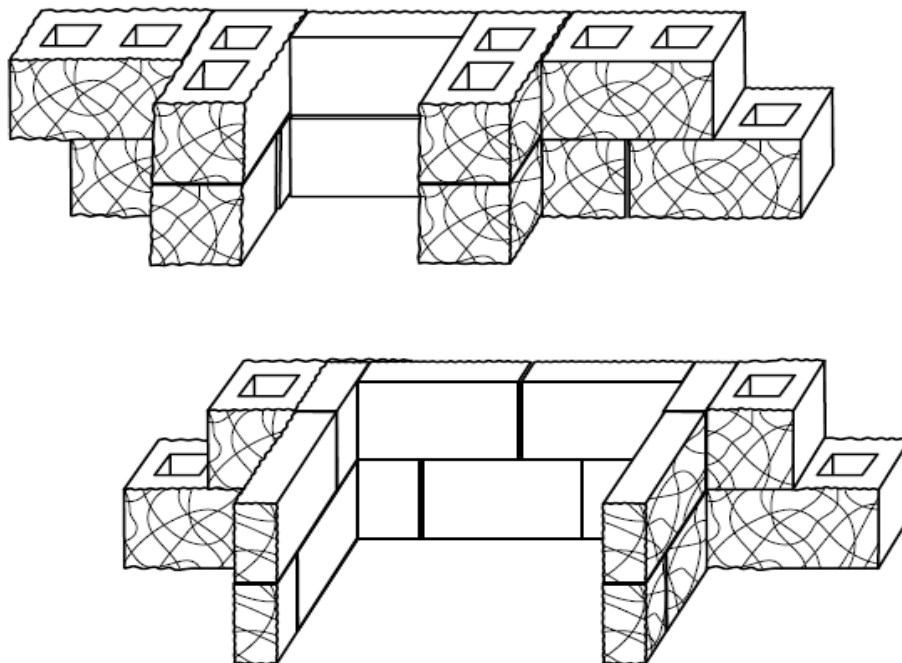
Obr. č.24 Nika pro plynoměr, elektroměr
