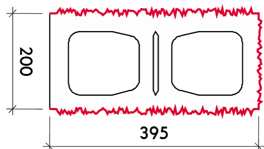
Obr. č.15 Okrasná tvárnice trojstranná D2
