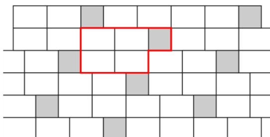
Obr. č.9 – Návrh pokládky z prvků Břidlice 60x40 a Břidlice 40x40
