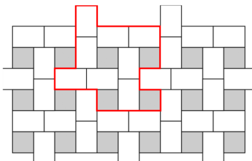
Obr. č.7 – Návrh pokládky z prvků Břidlice 60x40 a Břidlice 40x40
