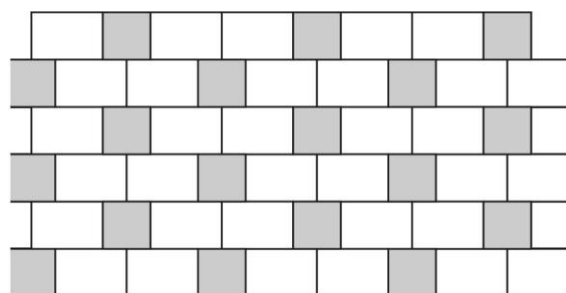
Obr. č.8 – Návrh pokládky z prvků Břidlice 60x40 a Břidlice 40x40
