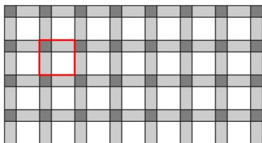
Obr. č.7 – Návrh pokládky z prvků Pl. Dlažba 40x40, Dekorační kostka 19,5x19,5 a Dekorační pás 40x19,5
