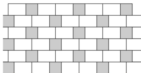
Obr. č.16 – Návrh pokládky z prvků Pl. Dlažba 60x40 a Pl. Dlažba 40x40
