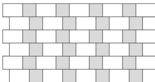
Obr. č.13 – Návrh pokládky z prvků Pl. Dlažba 60x40 a Pl. Dlažba 40x40
