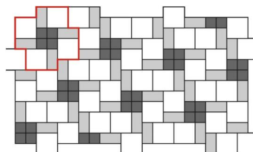
Obr. č.10 – Návrh pokládky z prvků Pl. Dlažba 40x40, Dekorační kostka 19,5x19,5 a Dekorační pás 40x19,5
