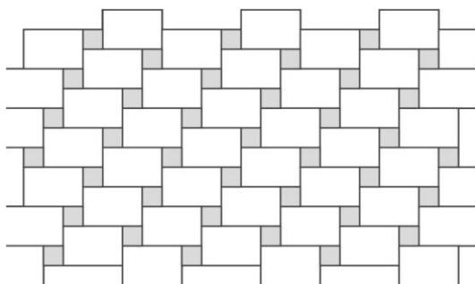
Obr. č.19 – Návrh pokládky z prvků Pl. Dlažba 60x40 a Dekorační kostka 19,5x19,5
