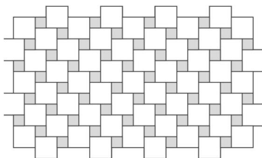
Obr. č.3 – Návrh pokládky z prvků Pl. Dlažba 40x40 a Dekorační kostka 19,5x19,5
