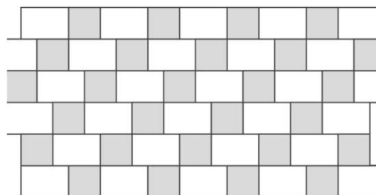
Obr. č.12 – Návrh pokládky z prvků Pl. Dlažba 60x40 a Pl. Dlažba 40x40
