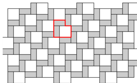
Obr. č.4 – Návrh pokládky z prvků Pl. Dlažba 40x40 a Dekorační pás 40x19,5
