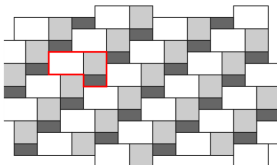
Obr. č.21 – Návrh pokládky z prvků Pl. Dlažba 60x40, Pl. Dlažba 40x40 a Dekorační pás 40x19,5
