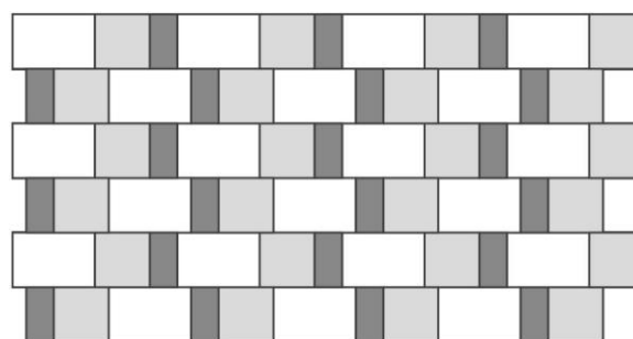
Obr. č.22 – Návrh pokládky z prvků Pl. Dlažba 60x40, Pl. Dlažba 40x40 a Dekorační pás 40x19,5
