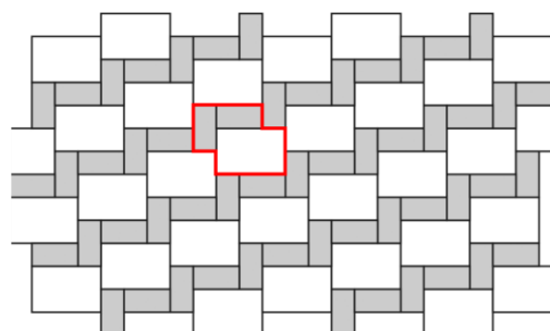
Obr. č.18 – Návrh pokládky z prvků Pl. Dlažba 60x40 a Dekorační pás 40x19,5
