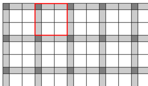
Obr. č.6 – Návrh pokládky z prvků Pl. Dlažba 40x40, Dekorační kostka 19,5x19,5 a Dekorační pás 40x19,5
