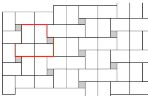
Obr. č.15 – Návrh pokládky z prvků Pl. Dlažba 60x40 a Dekorační kostka 19,5x19,5
