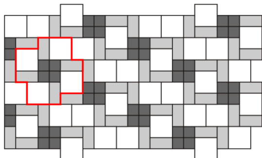
Obr. č.9 – Návrh pokládky z prvků Pl. Dlažba 40x40, Dekorační kostka 19,5x19,5 a Dekorační pás 40x19,5
