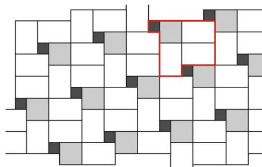
Obr. č.20 – Návrh pokládky z prvků Pl. Dlažba 60x40, Pl. Dlažba 40x40 a Dekorační kostka 19,5x19,5
