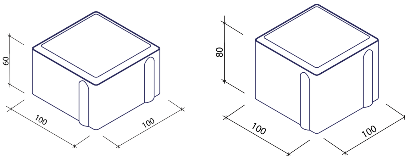
Obr. č.5- KOSTIČKA 6; 8 rozměry
