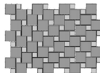
Obr. č.4 - Příklad pokládky betonové dlažby KOSTIČKA v kombinaci s KOSTKOU 200x200 mm
