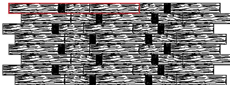
Obr. č.3 – Návrh pokládky z prvků Pražec - deska 60, Pražec - deska 120 a Pražec - špalek 15
