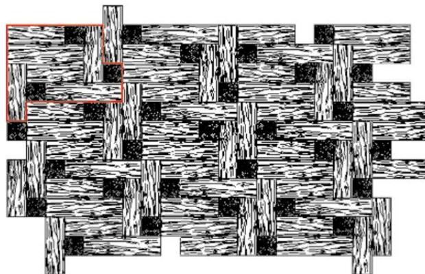
Obr. č.8 – Návrh pokládky z prvků Prkno I., prvků Prkno II. a Špalek
