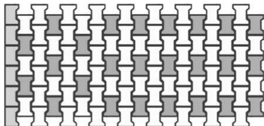
Obr. č.5 – Návrh pokládky z prvků Íčko a Íčko krajovka
