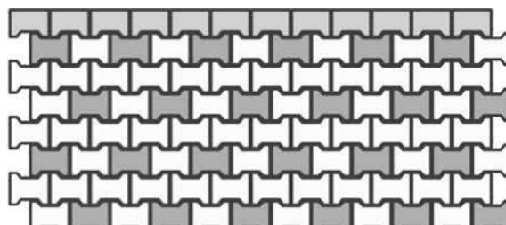
Obr. č.2 – Návrh pokládky z prvků Íčko a Íčko krajovka
