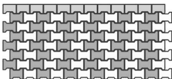
Obr. č.3 – Návrh pokládky z prvků Íčko a Íčko krajovka
