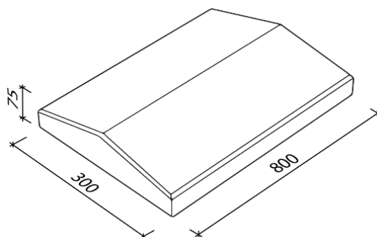
Obr. č.30 Zákrytová stříška 30 poloviční
