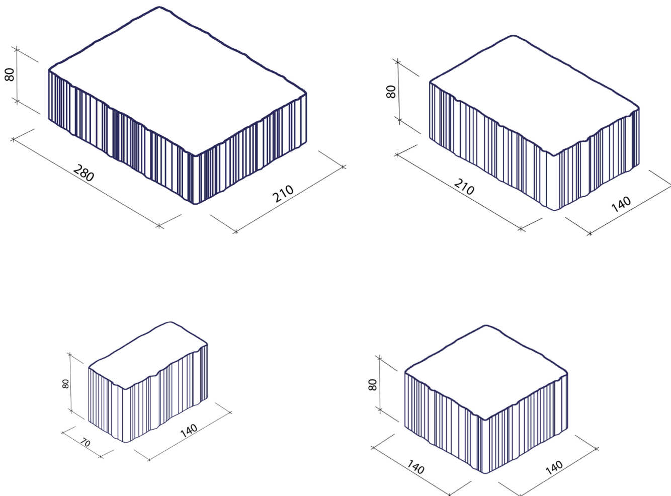
Obr. č.9 – MOZAIKA Rozměry kamenů
